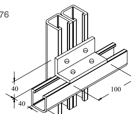
Junção Reta 90°
